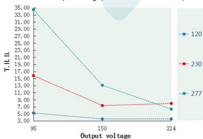
T.H.D. VS Output voltage(DL-150W-V214DX-MXG)
