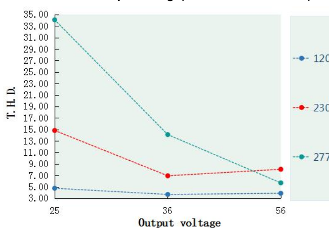
T.H.D. VS Output voltage(DL-150W-V56DX-MXG)
